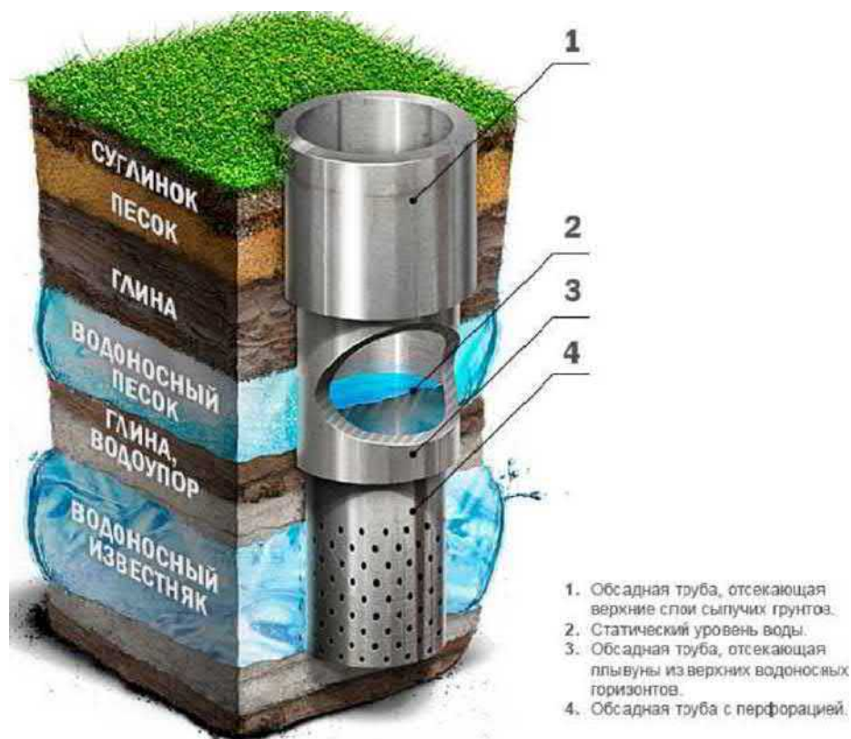
Рис. Конструкция артезианской скважины
